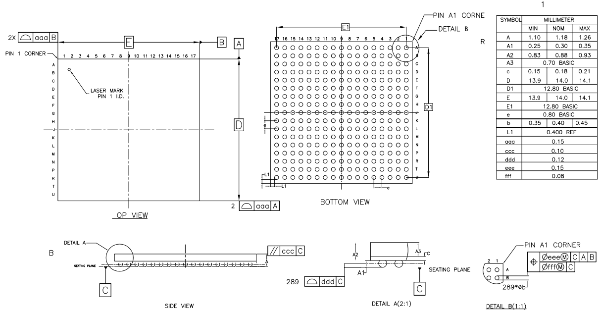
图 29: 289BGA 封装尺寸图
