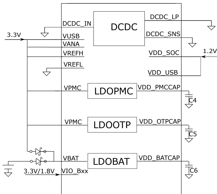
图 5: 不使用内置 DCDC 的系统供电框图
