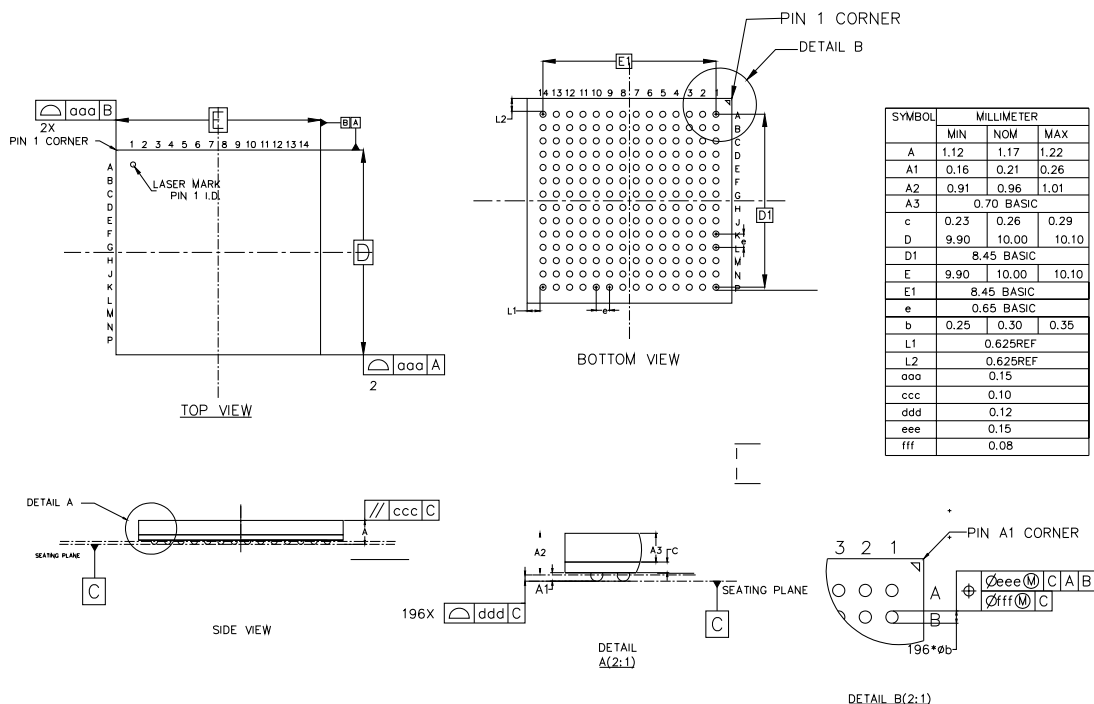
图 30: 196BGA 封装尺寸图
