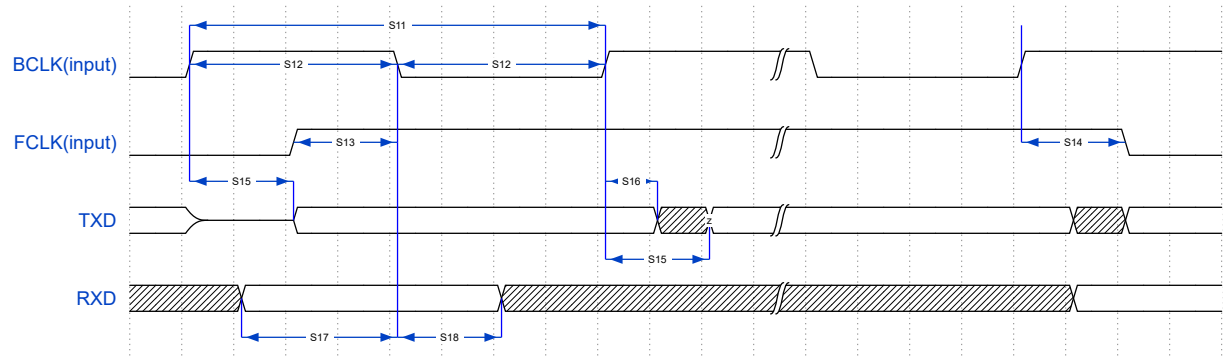
图 20: I2S 输入时钟时（TXD 数据在 BCLK 上升沿发出，RXD 在 BCLK 下降沿采样）
