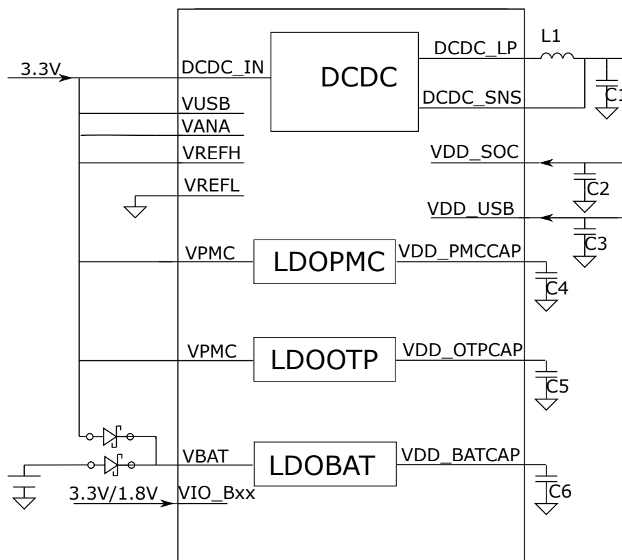
图 4: 使用内置 DCDC 的系统供电框图
